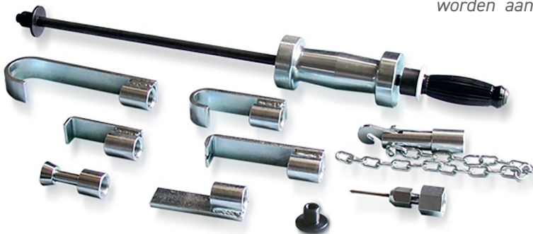
Slagtrekkerset 4Kg + 8 hulpstukken
